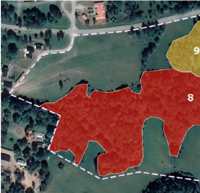
Karta över detaljerad inventering. EnviroPlanning (2021). Planområdet för vårdboendet bedöms enbart påverka naturområdets norra kant då det införlivas i vårdboendetomten.
